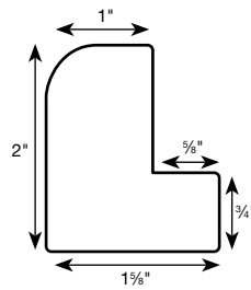
2" Bullnose L-Frame
