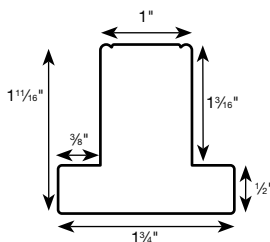
Deco T-Post
