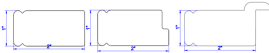
2" Butt Stile
