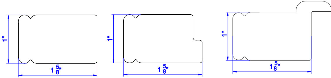
1 5/8" Butt Stile
