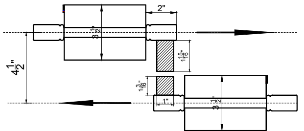
3 ½" Louver
