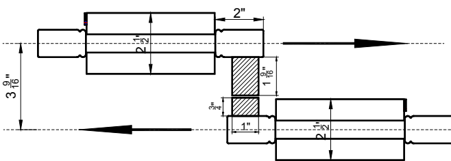
2 ½" Louver
