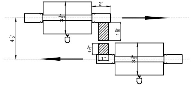
3 ½" Louver
