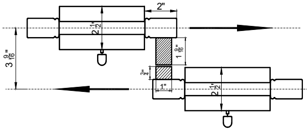
2 ½" Louver
